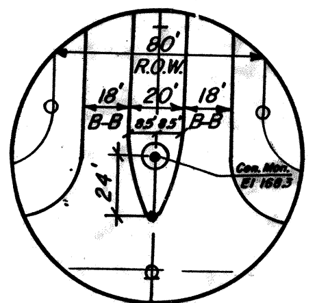
DETAIL N.T.S.
