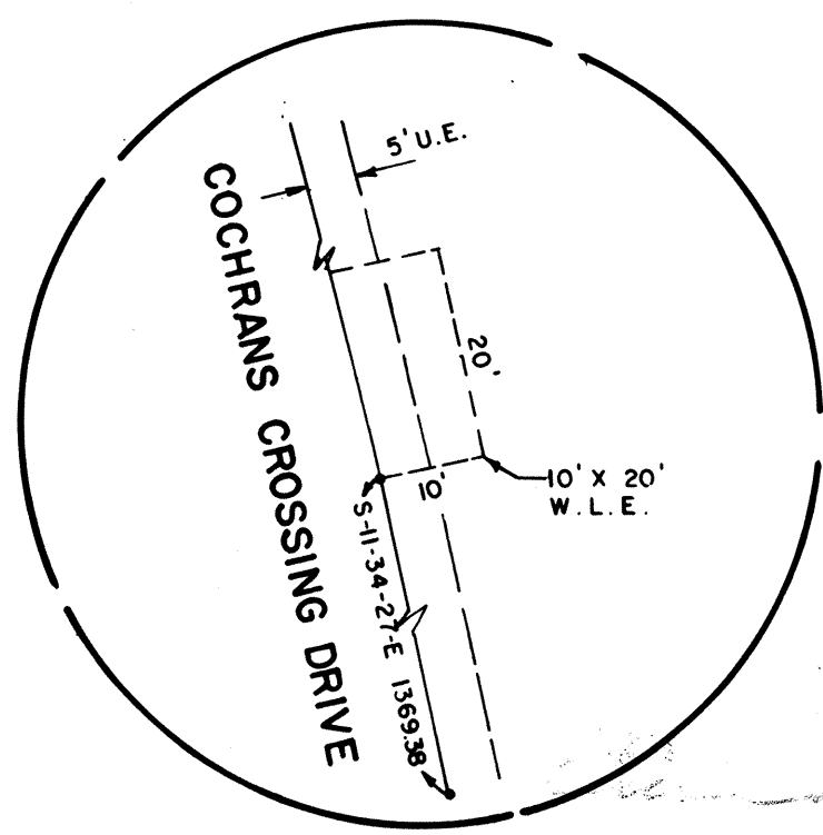
INSET "A" SCALE: 1" = 20'
